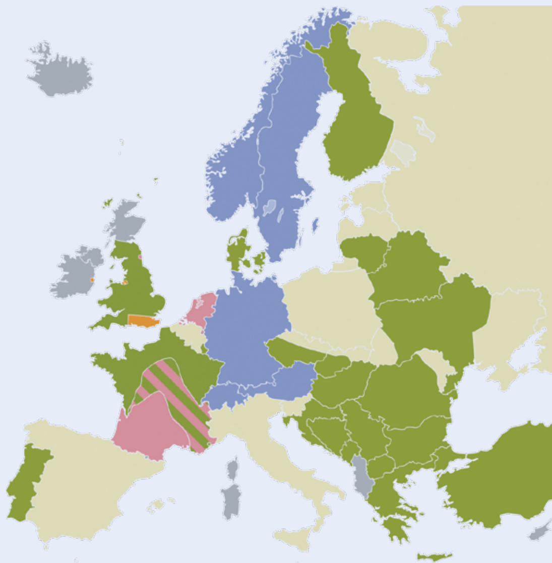
Főbb vasútvillamosítási rendszerek Európában: 750 V DC 15 kV AC 3 kV DC 1,5 kV DC 25 kV AC nincs villamosított vonal
